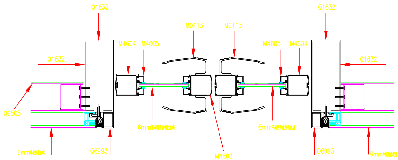
武汉学院实训楼幕墙JD-01
