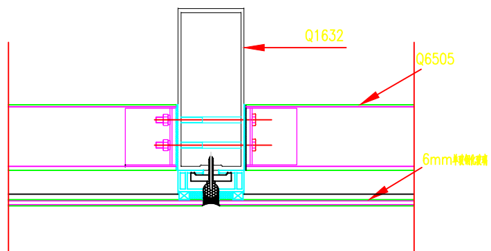
武汉学院实训楼幕墙JD-02
