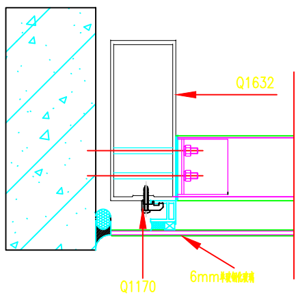
武汉学院实训楼幕墙JD-01
