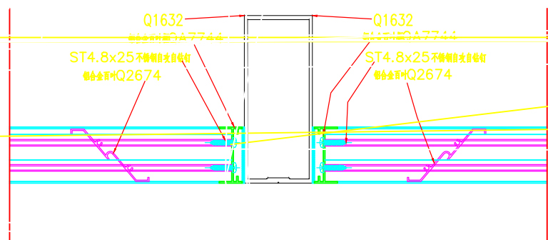
式样窗尖洞幕墙JD-07
